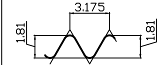
牙型和尺寸图
